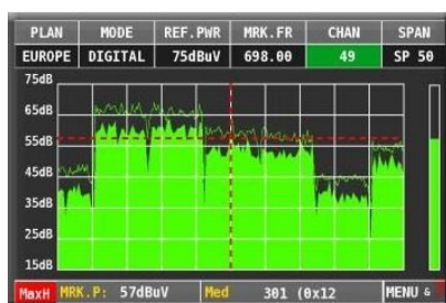
SPEKTRUM TV
