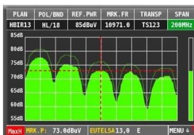
SPEKTRUM SAT
