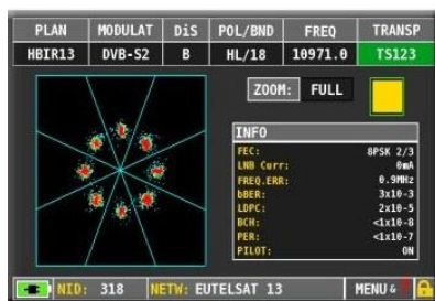
KONSTELACJA DVB-S2
